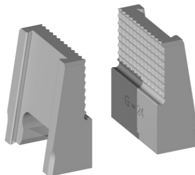
Ganasce zigrinate RC G=24 Nr. 835802
