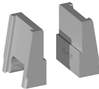
Ganasce a gradino RC G=24 Nr. 835480
