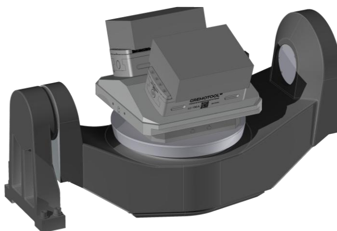
2x LC-150k (corto) con Prisma & System 3R Delphin 398 Pallet
