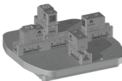
2x RC-38 rivolto verso l'esterno & System 3R Dynafix Pallet
