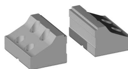
Ganasce di presa unilaterale alta
