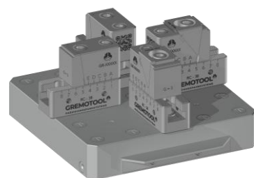
2x RC-38 rivolto verso l'esterno & System 3R GPS-240 Pallet
