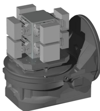
Ganascia: 8x 837150-B60 Dispositivo di serraggio: 8x LC-60
