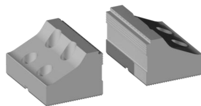
Ganascia di presa alta unilaterale
