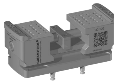
SC-120 & Erowa coni VPC 96
