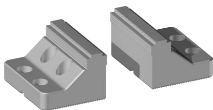
Ganasce di presa alte
