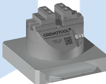
PMC-60 auf Palette
