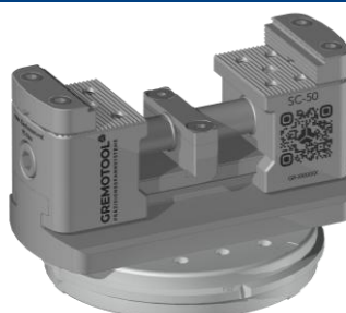
SC-50 mit System 3R GPS-120 Palette
