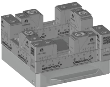
4x RC-38 mit System 3R GPS-240 Palette
