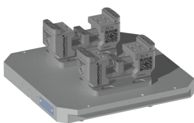
2x SC-74 mit System 3R Delphin 398 Palette
