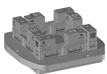
4x RC-38 mit System 3R Dynafix Palette
