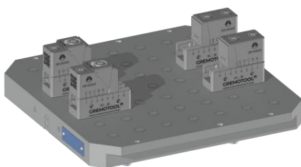
2x RC-38 mit System 3R Delphin 398 Palette
