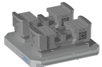
2x SC-120 mit System 3R Delphin 398 Palette
